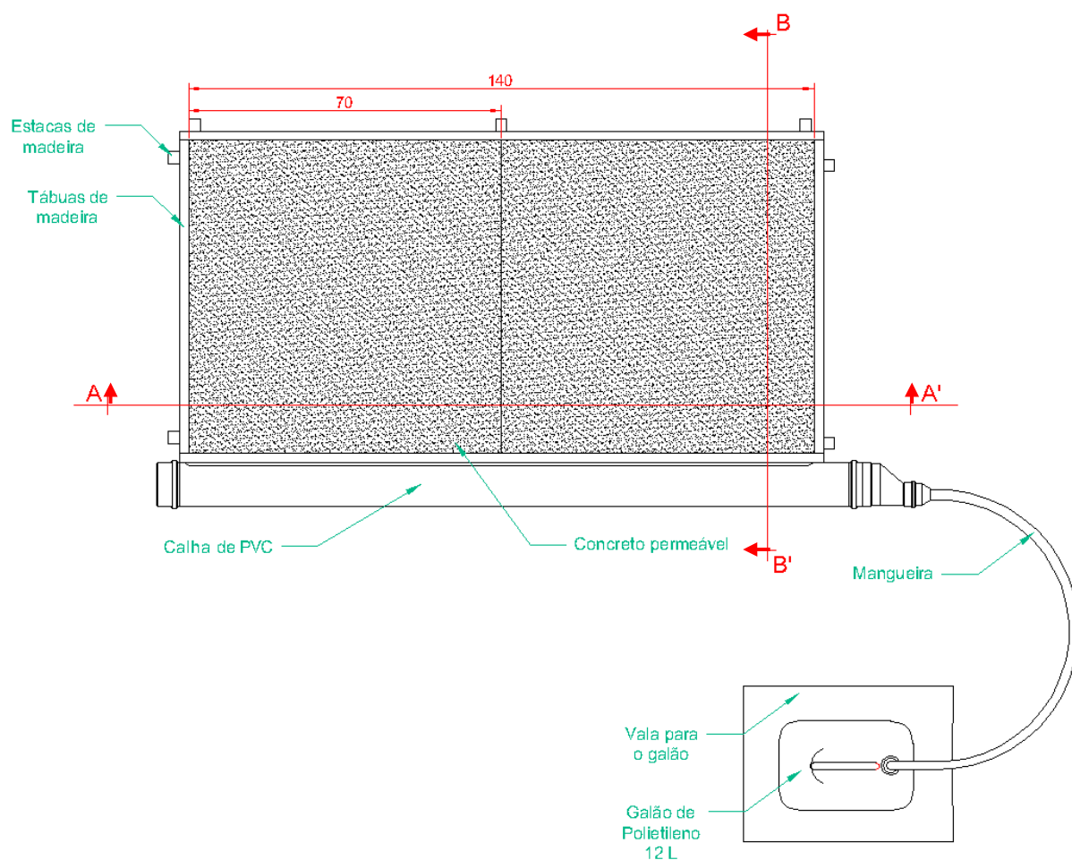
Figura 6. Planta baixa do modelo de pavimento de concreto permeável, com medidas em centímetros
