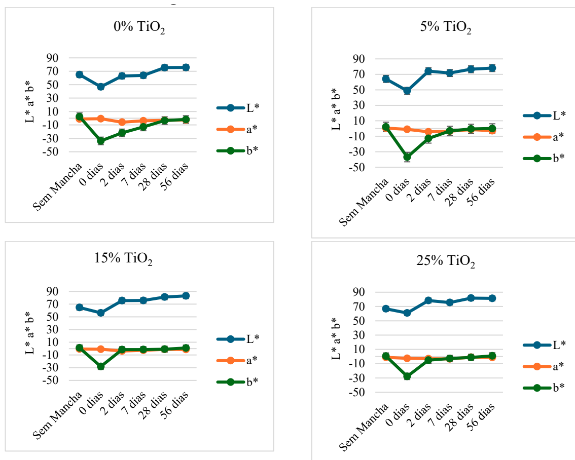
Figura 09. Resultados do sistema L^*a^*b^*
