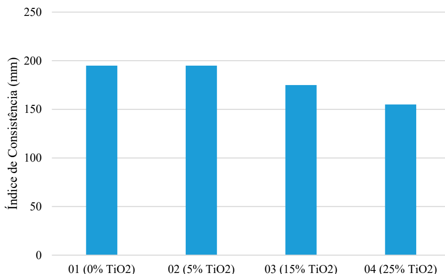
Figura 06. Resultados do índice de consistência
