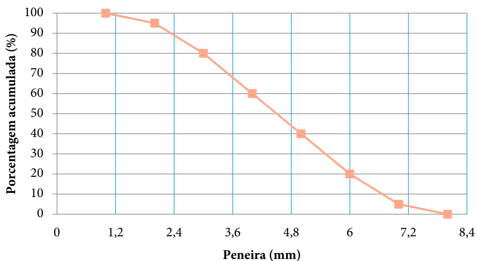
Figura 01. Curva de distribuição granulométrica da areia
